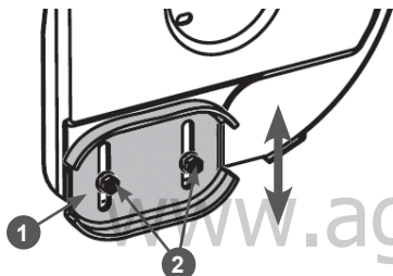
Рис. 29 Регулировка высоты забора снега 1. Полозок 2. Гайка (2 шт.)
