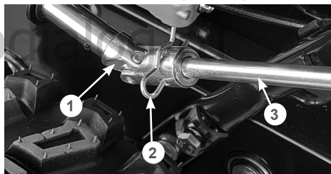
Рис. 27 Крепление рычага управления поворотом жёлоба
