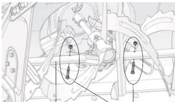
Ось шнека
