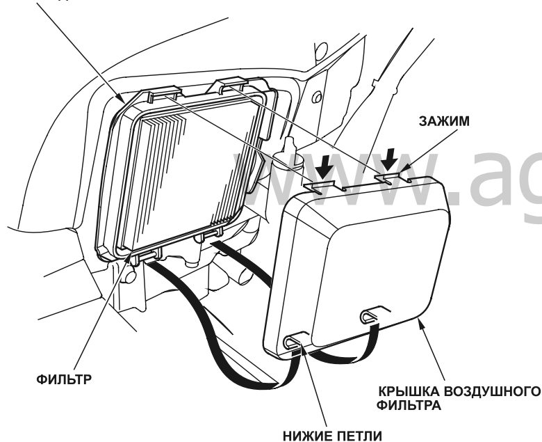
КОРПУС ВОЗДУШНОГО ФИЛЬТРА
