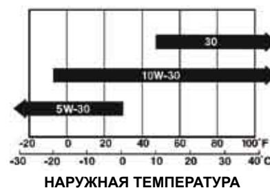
SAE Степени вязкости
