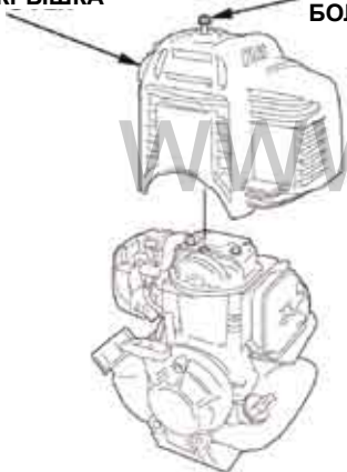
ВЕРХНЯЯ КРЫШКА 5 мм ШЕСТИГРАННЫЙ БОЛТ
