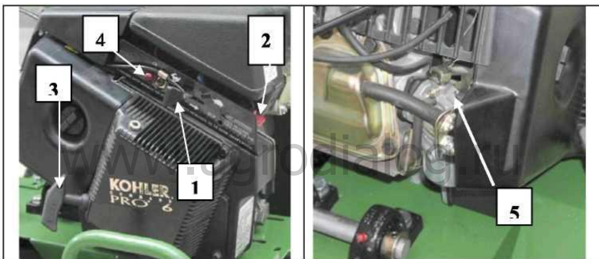
Органы управления на двигателе
