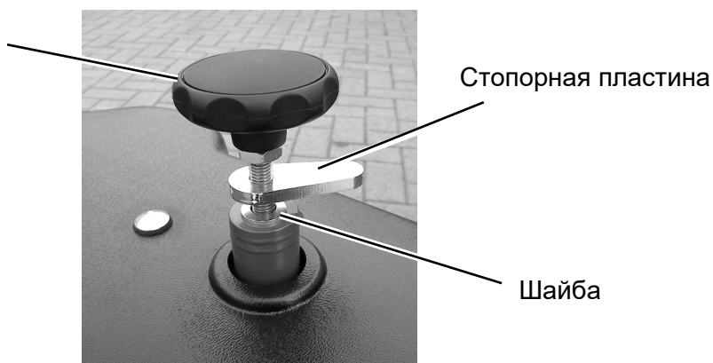
Рисунок 8: Винт с барашком для регулировки щетки по высоте
