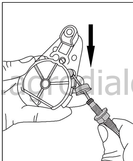
Рис. 21. Установка тросика
