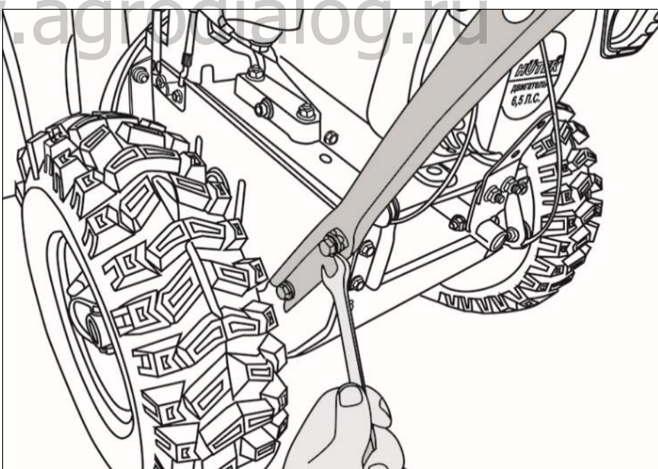
Рис. 4. Закрепление рукоятки управления на раме
