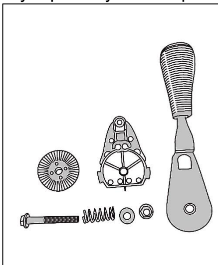
Рис. 19. Рукоятка переключения передач
