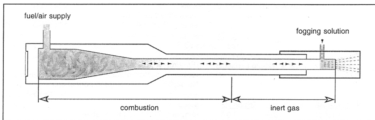
Рис.1.Камера сгорания и резонатор.
