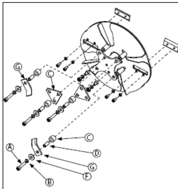
РИСУНОК 14 – Корпус ротора
