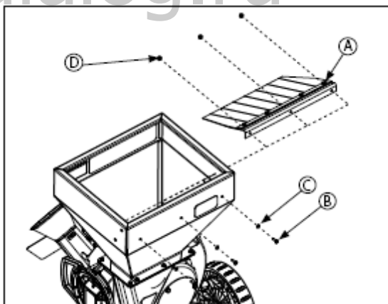
РИСУНОК 4 – Установка кожуха лотка измельчителя
