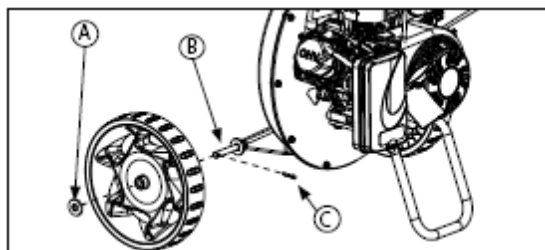
РИСУНОК 2 – Установка колес
