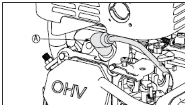
РИСУНОК 12 А. Защитный колпачок / провод свечи зажигания
