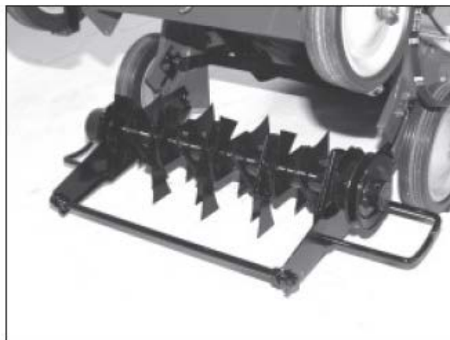
2) Подвижные ножи
