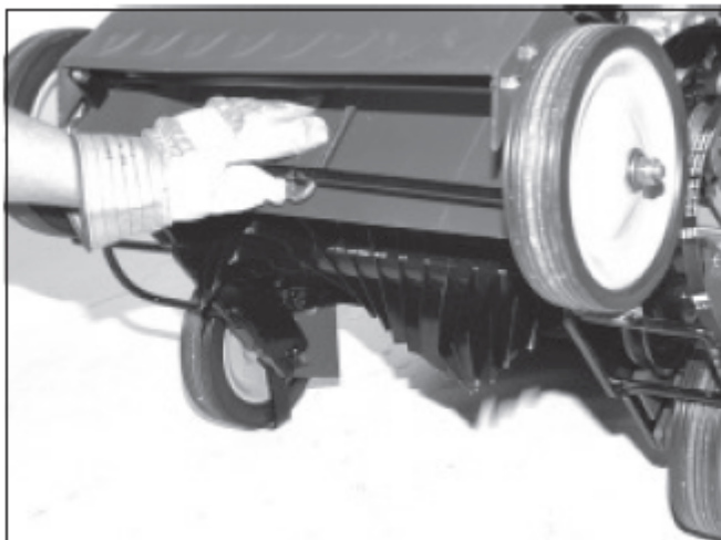
3) Приподнять узел скарификатора и навесить на крючки
