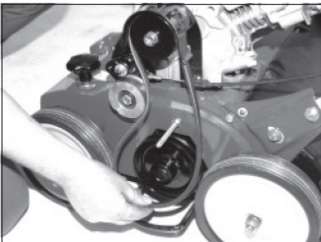
7) Затем поставить скарификатор на колеса и наложить клиновой ремень.
